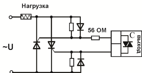
Подключение внешних тиристоров
