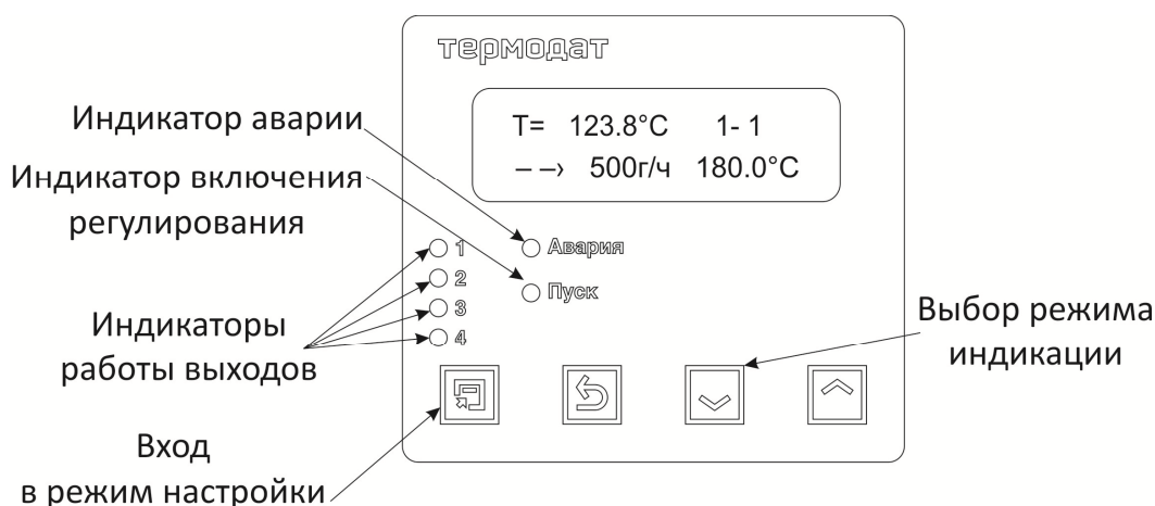
Рисунок 2 – Описание индикаторов и кнопок управления прибора
