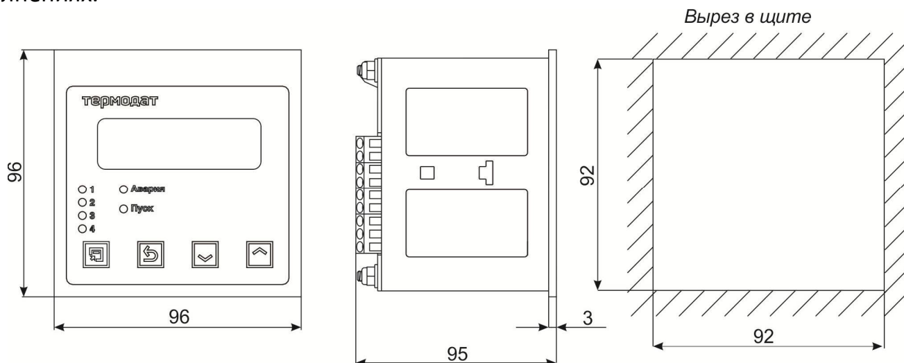
Рисунок 11 – Габаритные размеры прибора 14E5/...../ или Термодат-14E5-A
