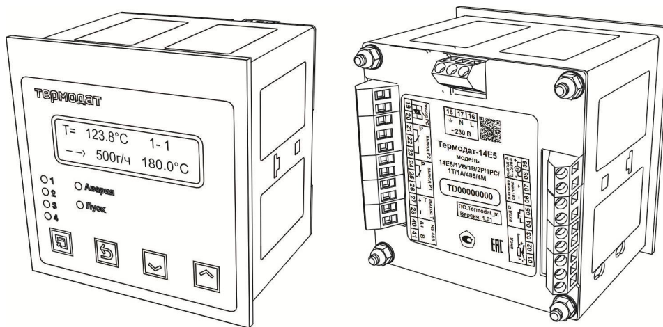
Рисунок 1 – Внешний вид прибора Термодат-14Е5
