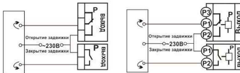
Рисунок 6 – Схемы подключения релейных выходов
