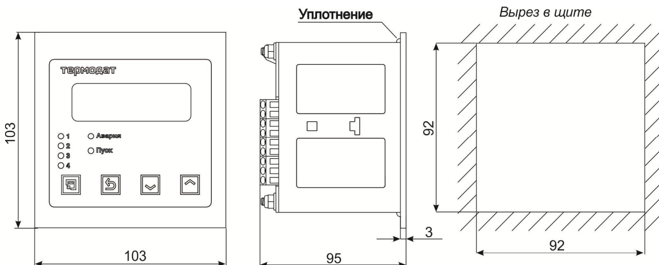
Рисунок 12 – Габаритные размеры прибора Термодат-14E5/...../IP67пп или Термодат-14E5-A7
