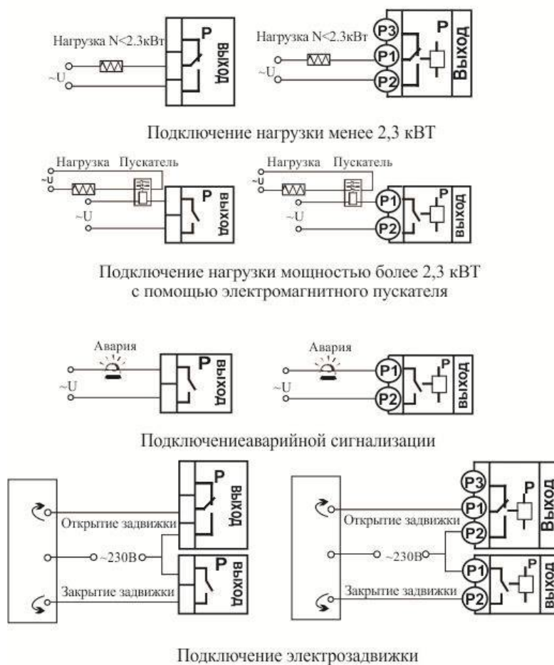
Рисунок 6 – Схемы подключения релейных выходов
