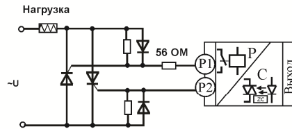
Подключение внешних тиристоров
