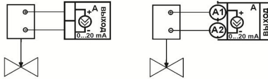
Подключение задвижки с электроприводом
