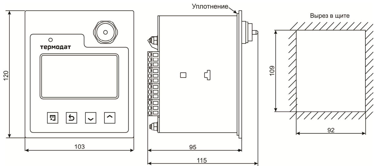
Рисунок 12 – Габаритные размеры прибора Термодат-16К6/...../IP67пп или Термодат-16К6-А7
