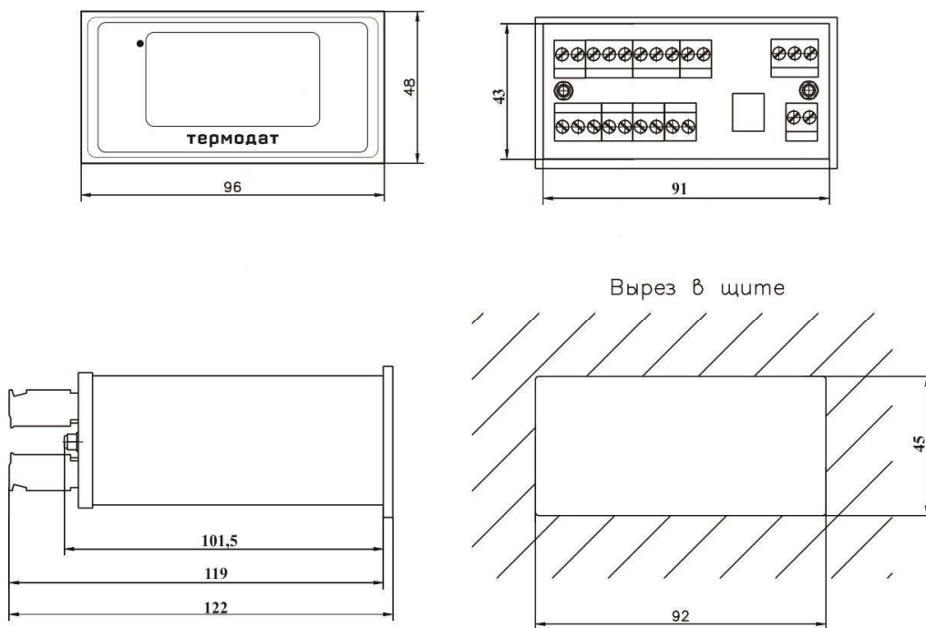
Рисунок 14 – Габаритные размеры прибора Термодат-16Е6-Н-(F)-(Eth)
