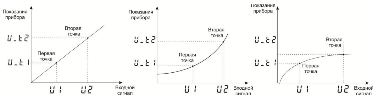
Рисунок 3 –Графики линейной, квадратичной зависимости или зависимости с извлечением квадратного корня для входа
