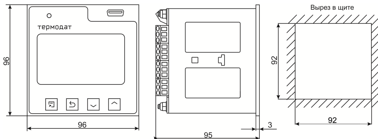
Рисунок 11 – Габаритные размеры прибора Термодат-16К6/...../(F) или Термодат-16К6-А-(F)-(Eth)
