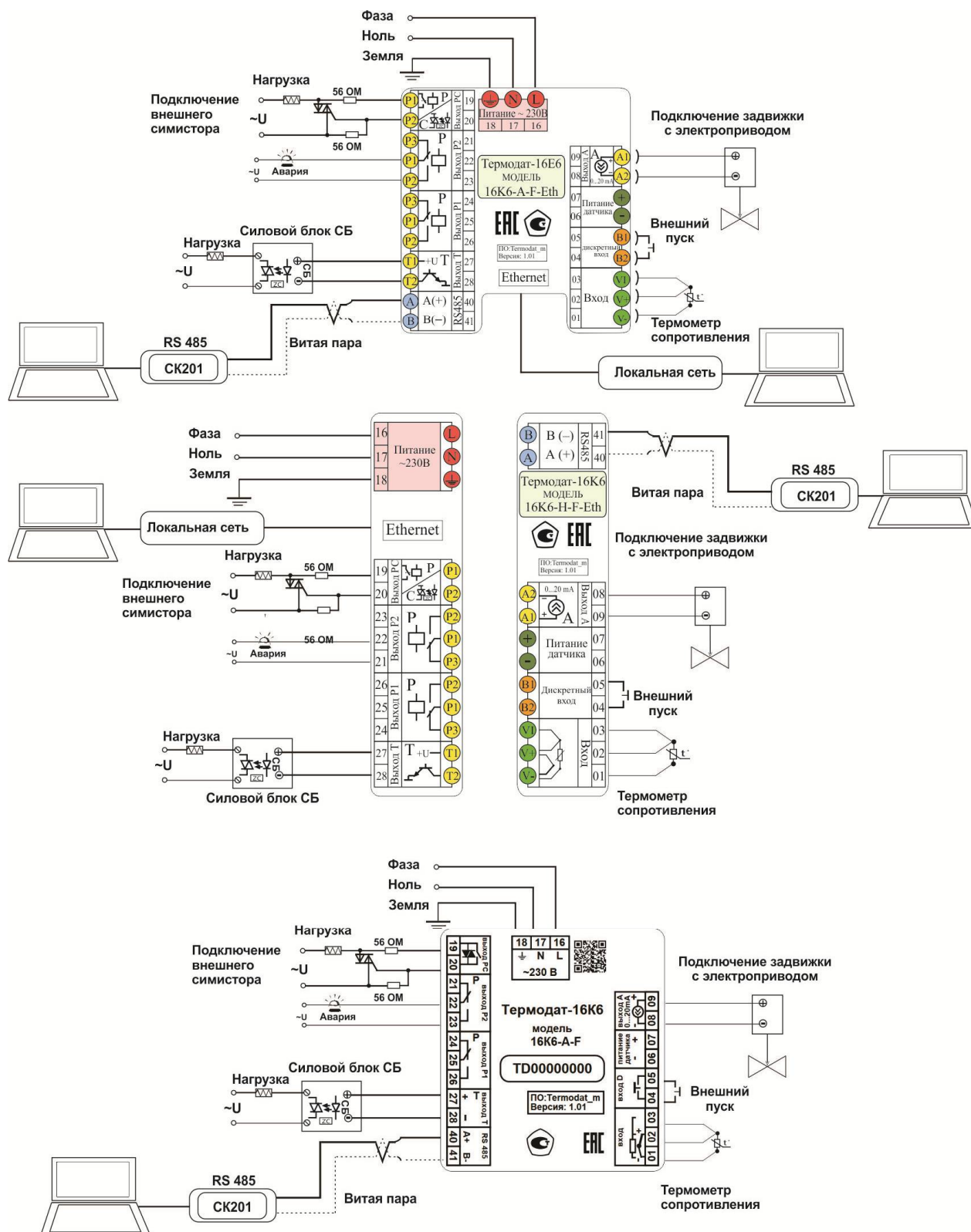
Рисунок 10 – Схема подключения прибора
