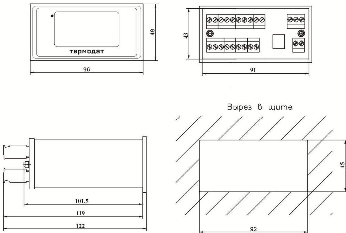
Рисунок 11- Габаритные размеры прибора Термодат-16М6/..../F/IP67пп или Термодат-16М6-А9-(F)
